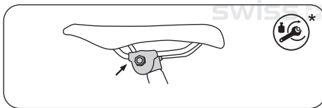
Befestigung mit Sattelkloben
