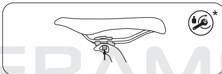
Patentstütze mit Einschraubenbefestigung
